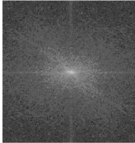
|F(u,v)|
