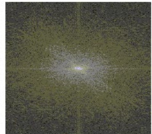
D(u,v)
